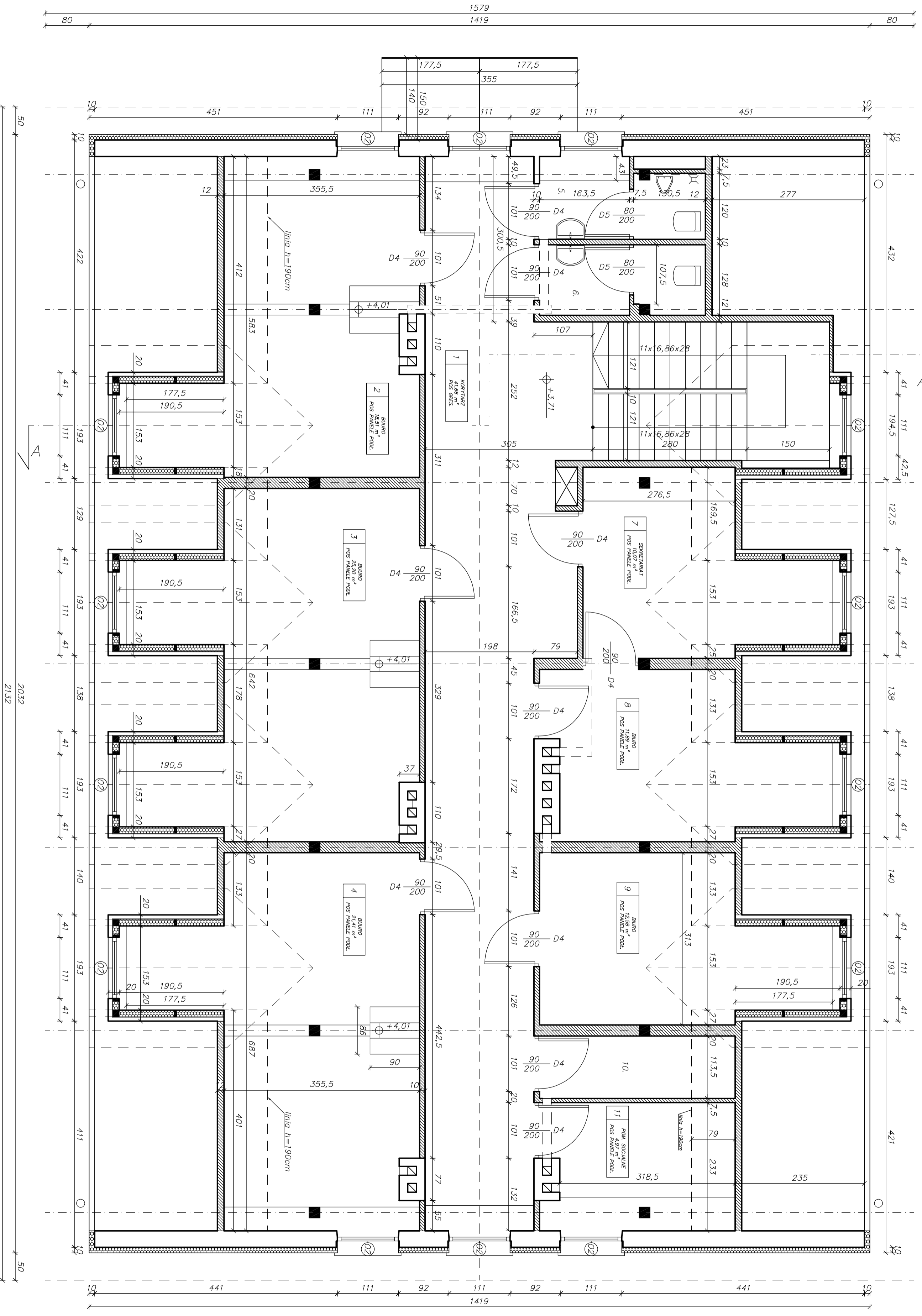
RZUT PODDASZA SKALA 1:50
